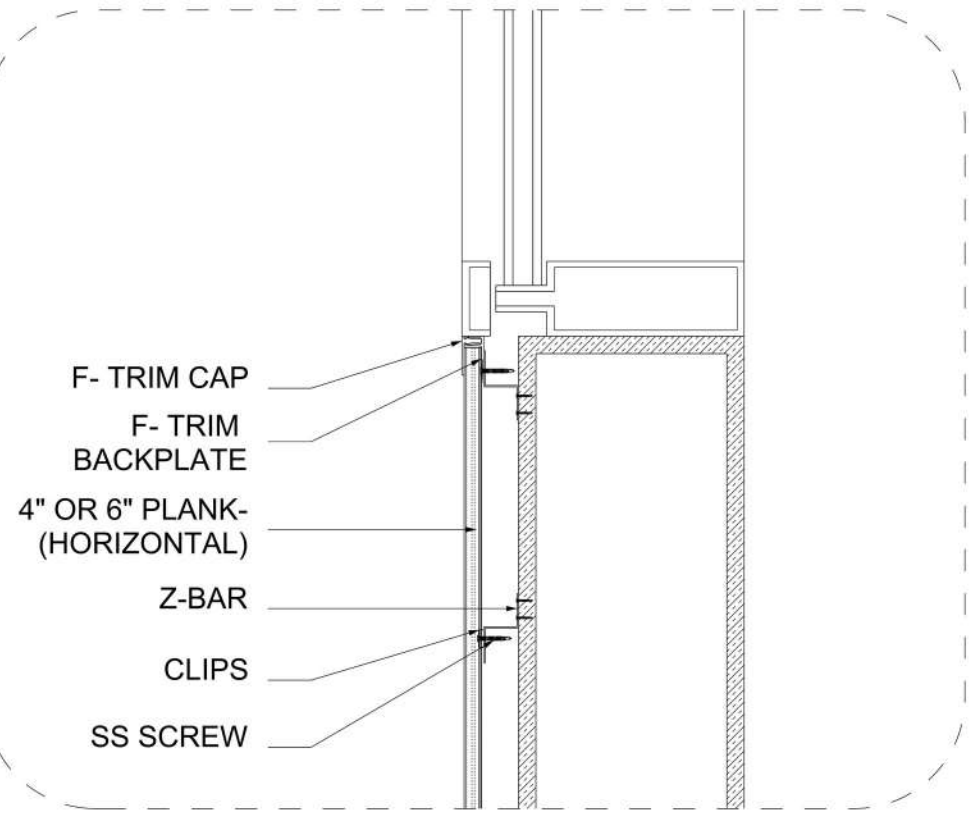
D DETAIL D-08 SCALE: 1.0" 2.0" 5.0"
