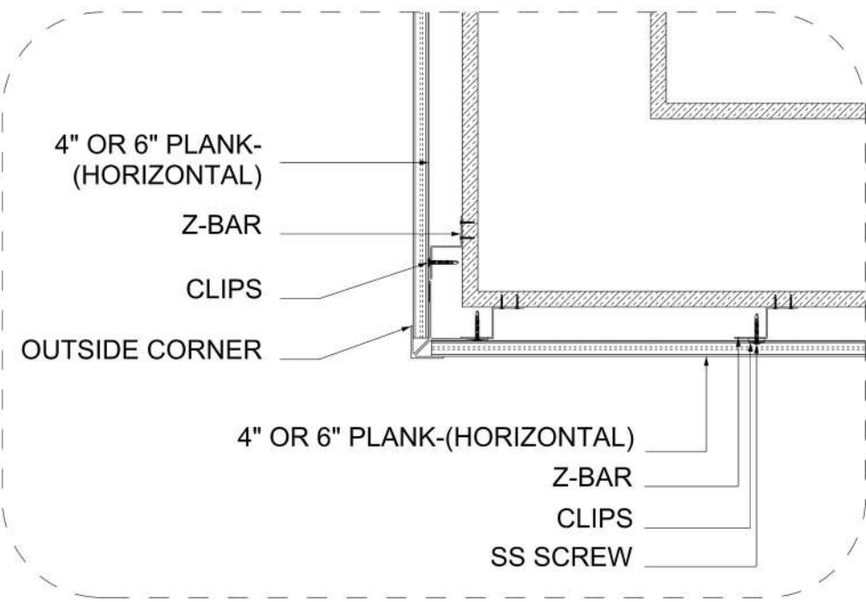
D DETAIL D-09 SCALE: 1.0" 2.0" 5.0"
