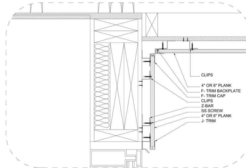
D DETAIL S-08 SCALE: 1.0" 2.0" 5.0"
