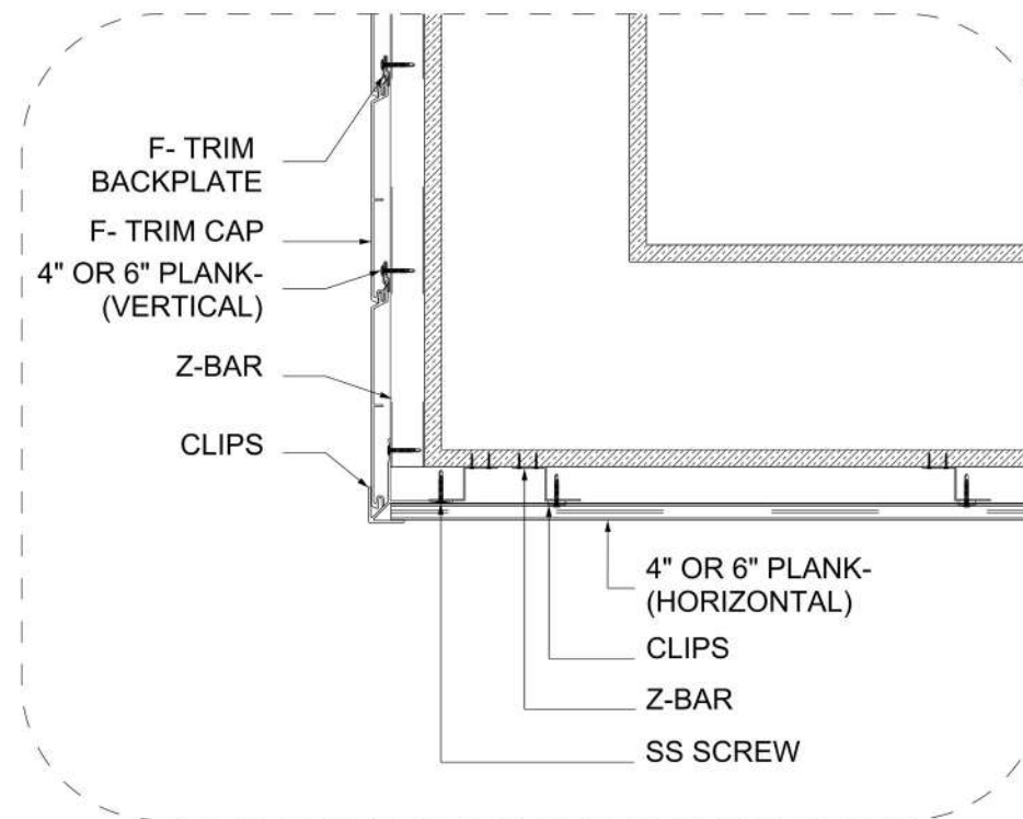
D DETAIL D-06 SCALE:
