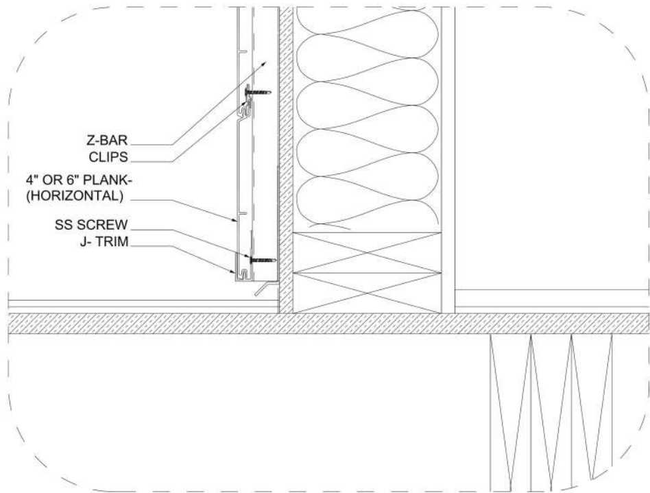
D ETAIL S-04
