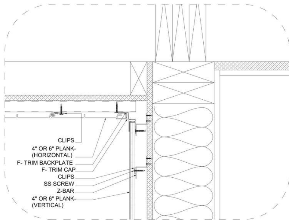
D ETAIL S-05
