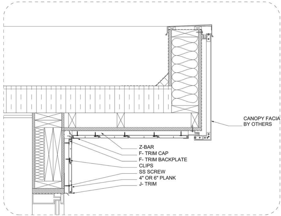
D DETAIL S-07 SCALE: 1.0" 2.0" 5.0"
