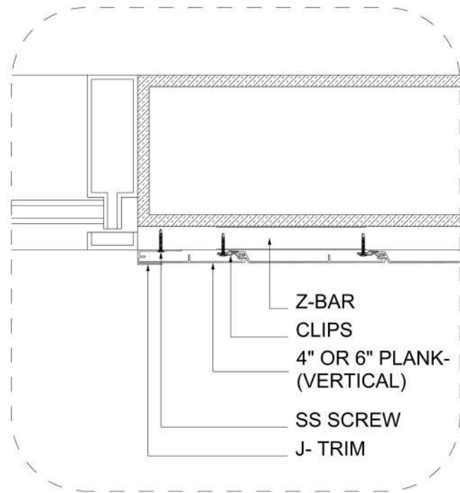
D DETAIL D-04 SCALE:
