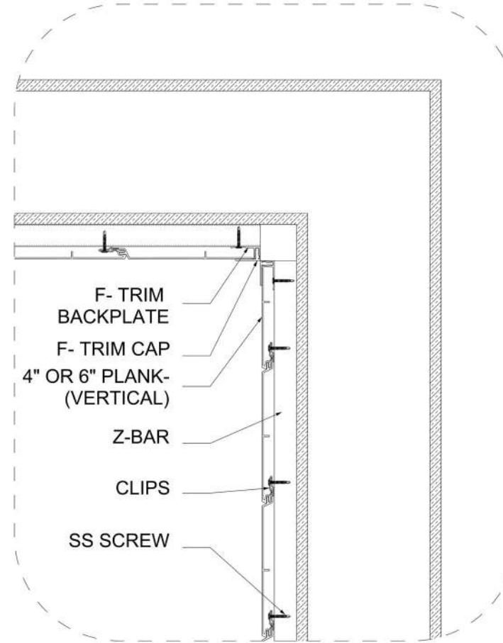
D DETAIL D-05 SCALE:
