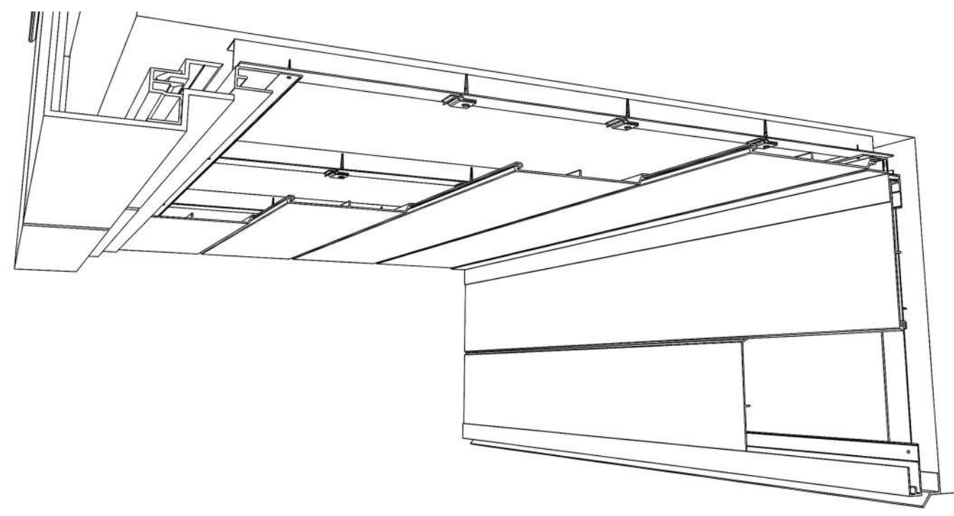
D DETAIL S-01 SCALE: 1.0" 2.0" 5.0"
