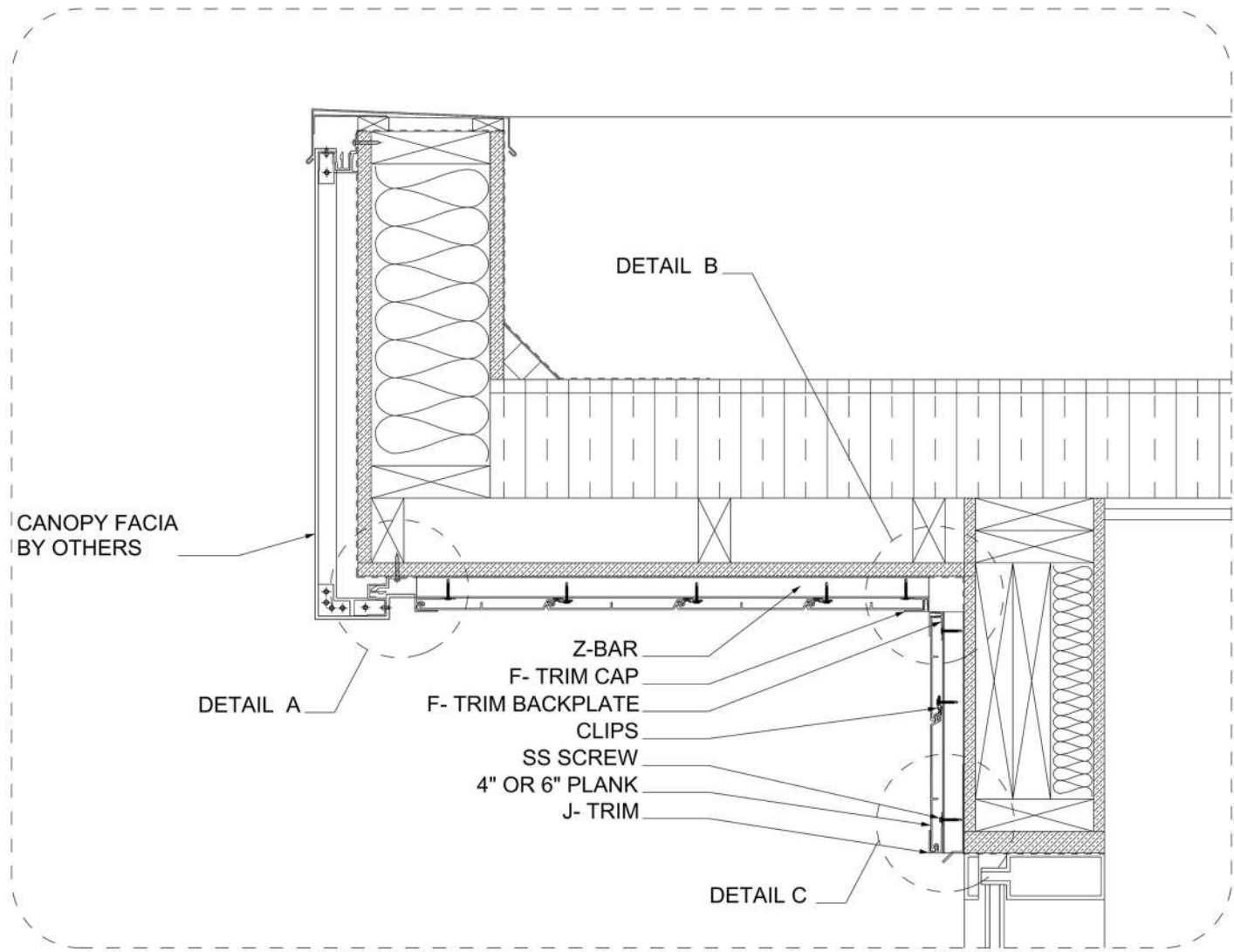
D DETAIL S-01 SCALE: 1.0" 2.0" 5.0"
